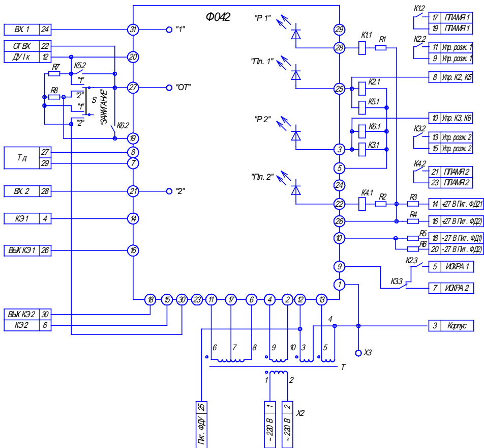
Рисунок 3 - Схема электрическая прибора Ф34.2
