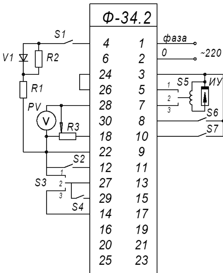
Рисунок 7 - Схема проверки прибора Ф34.2
