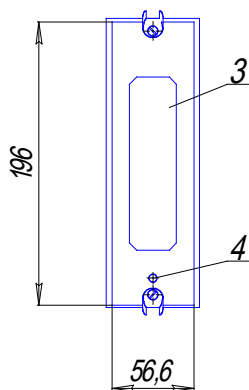
Рисунок 1 - Габаритные и установочные размеры прибора Ф34.2
