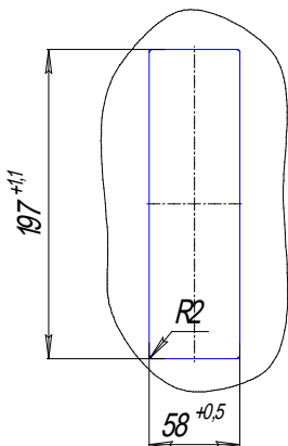
Рисунок 1 - Габаритные и установочные размеры прибора Ф34.2
