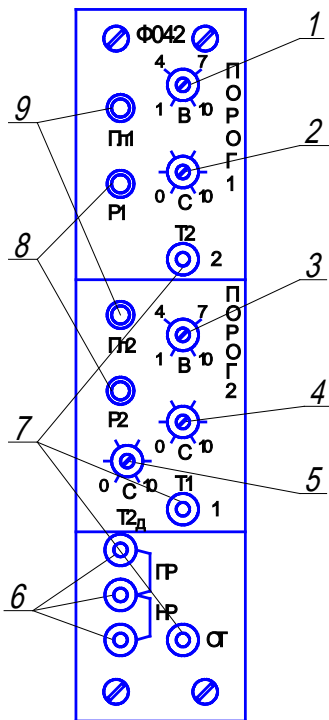
Рисунок 2 - Органы управления и контроля субблока Ф042
