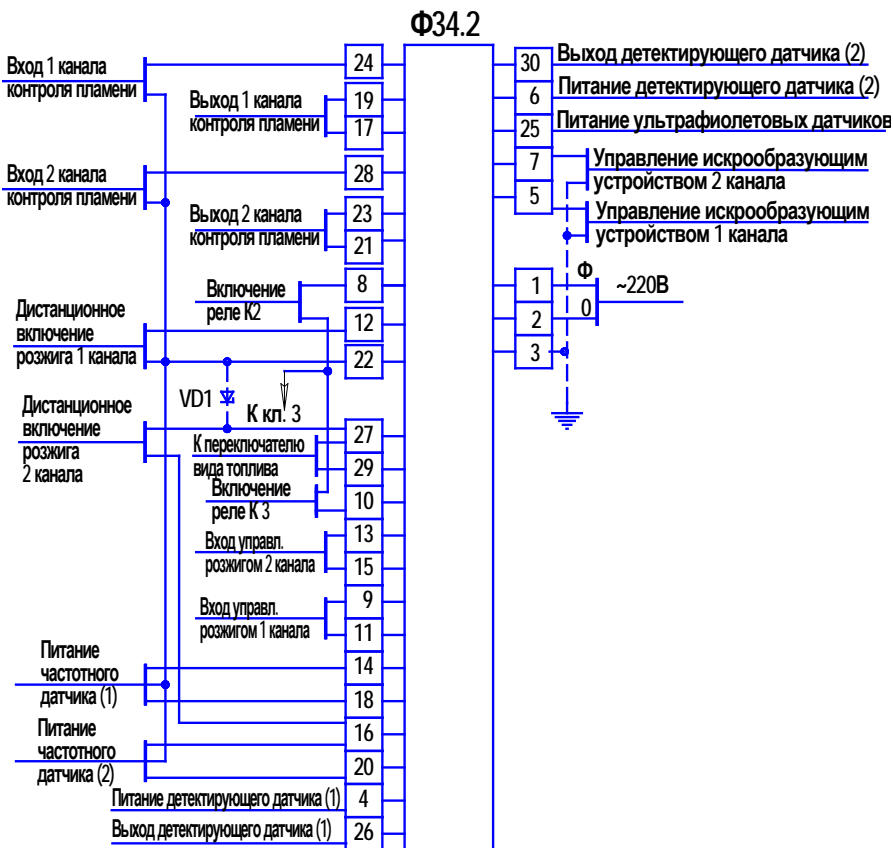
Рисунок 4 - Схема подключения прибора Ф34.2
