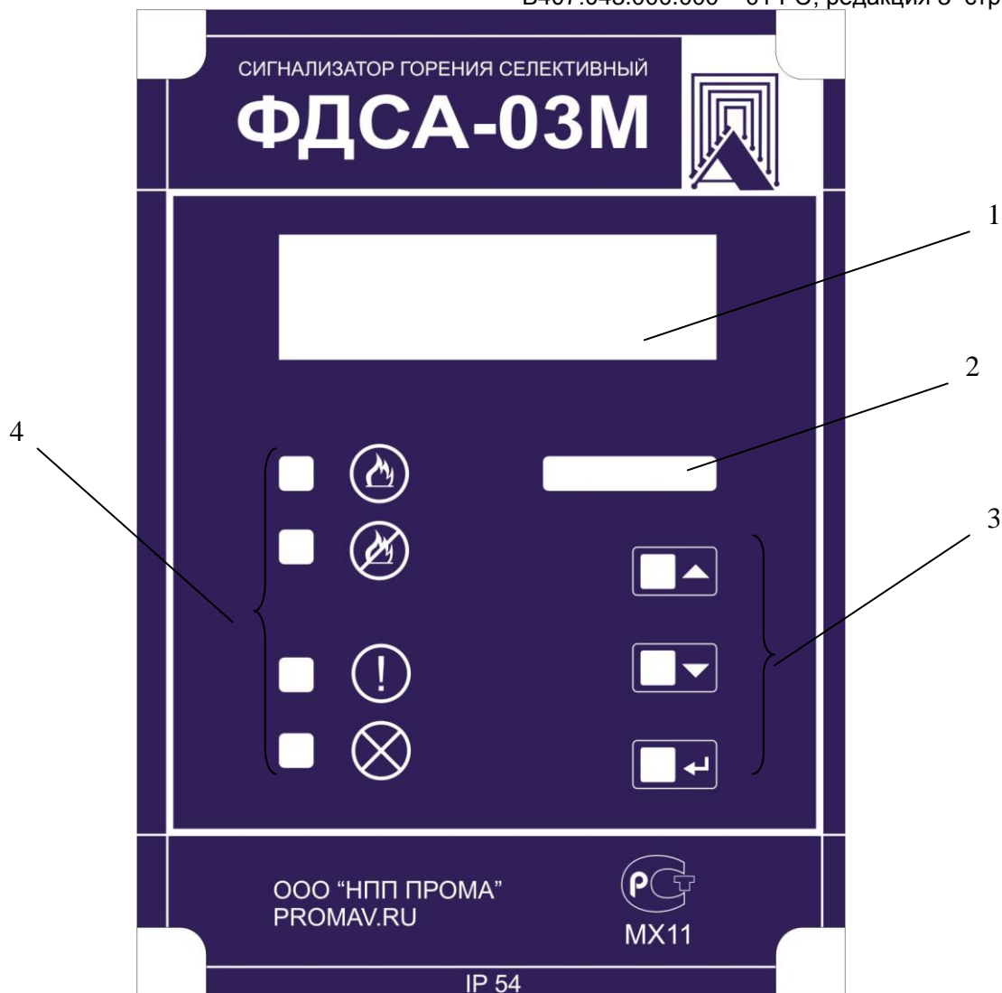
Рисунок 1. Лицевая панель устройства контроля пламени ФДСА-03М.
