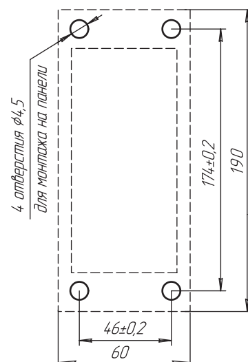
Разметка отверстий для крепления усилителя У29.3М
